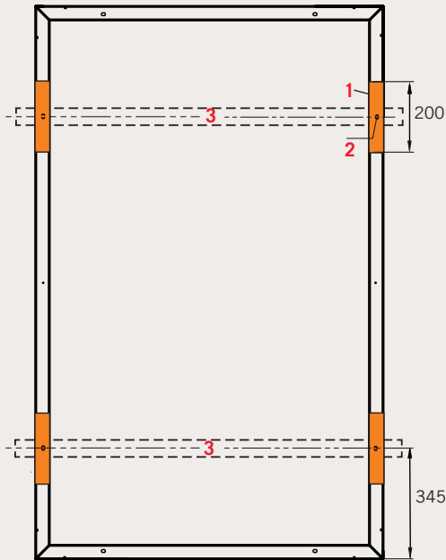
ABBILDUNG 2: Klemmbereiche für Schienenmontage quer in mm
