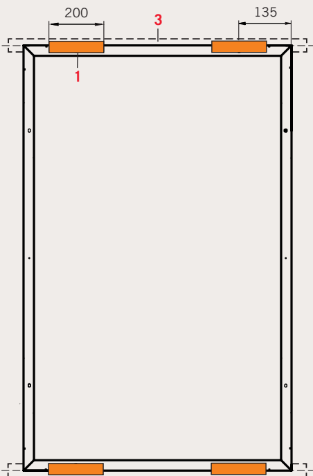
ABBILDUNG 4: Klemmbereiche für Einlegeprofile in mm
