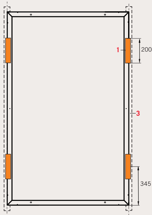
ABBILDUNG 3: Klemmbereiche für Schienenmontage längs in mm
